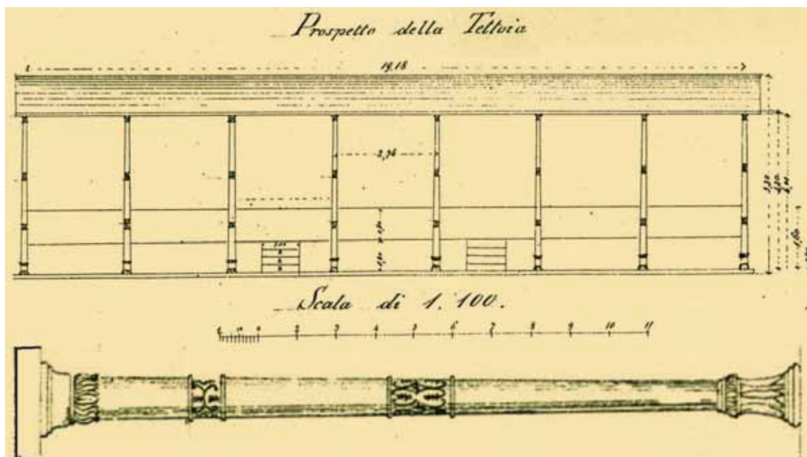
Prospetto della tettoia, disegnato dall'ingegner Olinto Citti di Pisa
