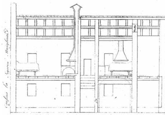
Particolari della nuova struttura, progettata dall'Ingegnere Costa
